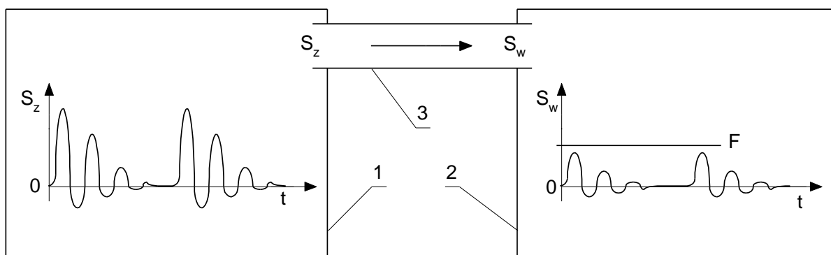
Rysunek 1. Szkic przedstawiający zjawisko sprzężenia elektromagnetycznego zakłócającego; 1 – obiekt zakłócający, 2 – obiekt zakłócany, 3 – droga przesyłu sygnału zakłócającego, F – dopuszczalny poziom zakłócenia, S_z – sygnał zakłócający, S_w – sygnał w obiekcie zakłócanym.
