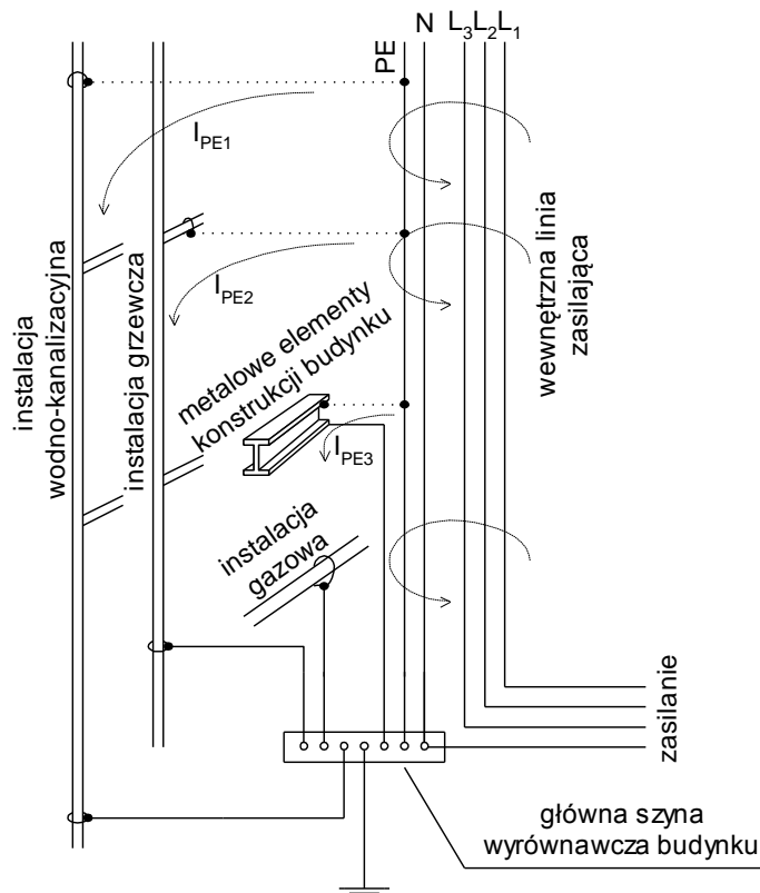
Rysunek 6. Szkic ilustrujący niekorzystny wpływ oddziaływań elektromagnetycznych na obciążenie przewodu PE w instalacji elektrycznej dużych obiektów budowlanych, wykonanej w systemie TN-S.
