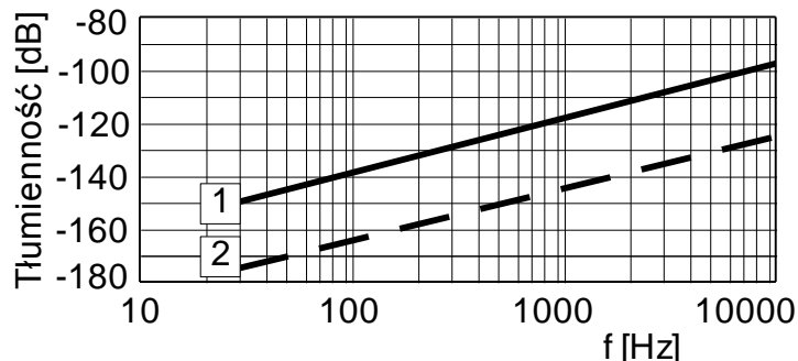
Rysunek 4. Tłumienność przenikowa przewodów pojedynczo ekranowanych w wiązce równoległej (1) i skrętej (2) w funkcji częstotliwości w zakresie od 30 Hz do 10 kHz.
