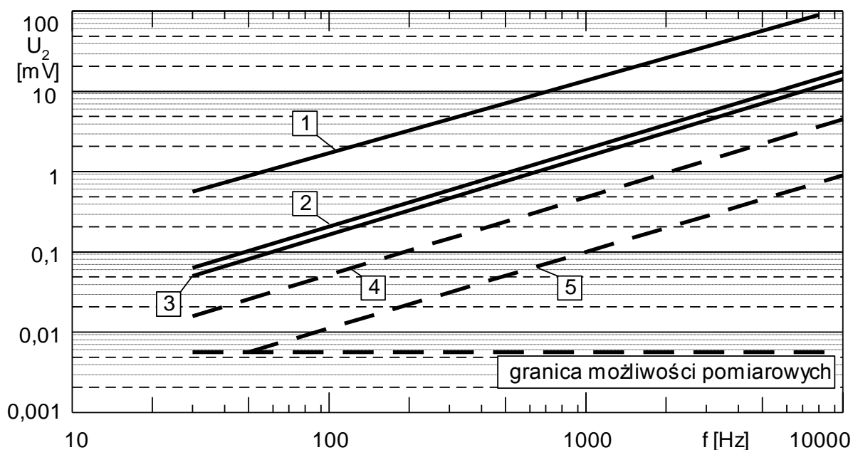
Rysunek 3. Przykładowe wartości napięcia indukowanego w próbkach przewodów instalacyjnych o długości 2m o dwóch różnych rodzajach prowadzenia wg [1]; 1 - wiązka równoległa, przewody nie ekranowane, 2 - wiązka równoległa, przewody ekranowane pojedynczo, 3 - wiązka równoległa, przewody ekranowane podwójnie, 4 - wiązka skrętna, przewody nie ekranowane, 5 - wiązka skrętna, przewody ekranowane pojedynczo.
