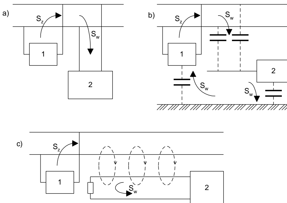
Rysunek 2. Przykłady sprzężeń zakłócających: a) galwaniczne, b) pojemnościowe, c) indukcyjne; oznaczenia jak na rys. 1.
