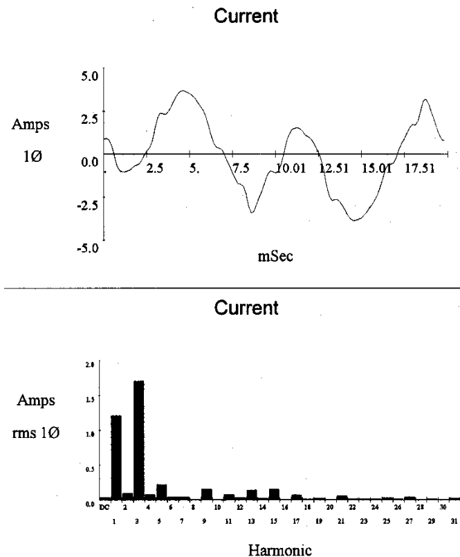
Rysunek 7. Przykładowy, typowy przebieg prądu w przewodzie PEN wraz ze spektrum wyższych harmonicznych.
