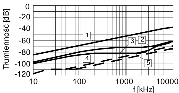
Rysunek 5. Tłumienność przenikowa przewodów instalacyjnych w funkcji częstotliwości w zakresie od 10 kHz do 10000 kHz; oznaczenia cyfrowe jak na rys. 3.
