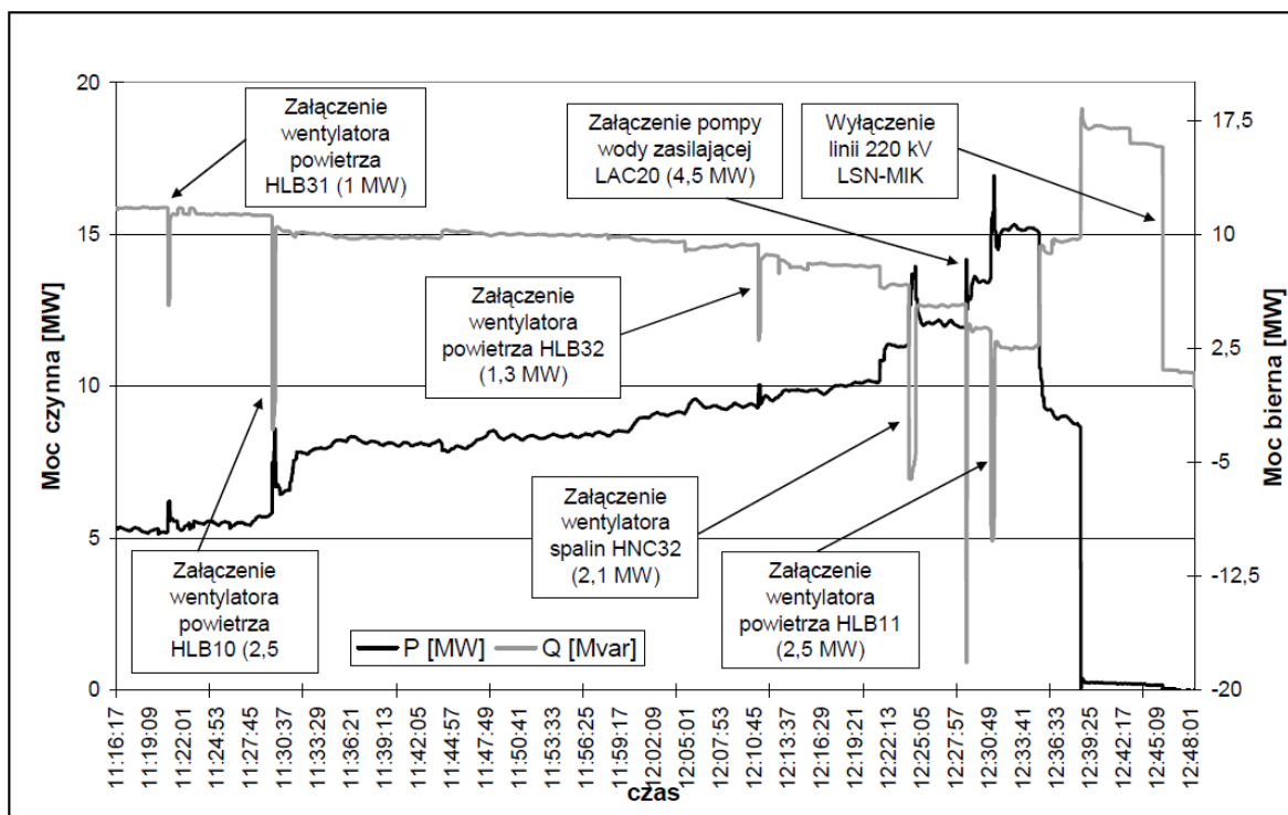
Rys. 10. Moc czynna i bierna w linii 110 kV kierunku Krosno Odrzańskie w czasie uruchamiania bloku energetycznego w El. Turów podczas eksperymentu w 2008 roku
