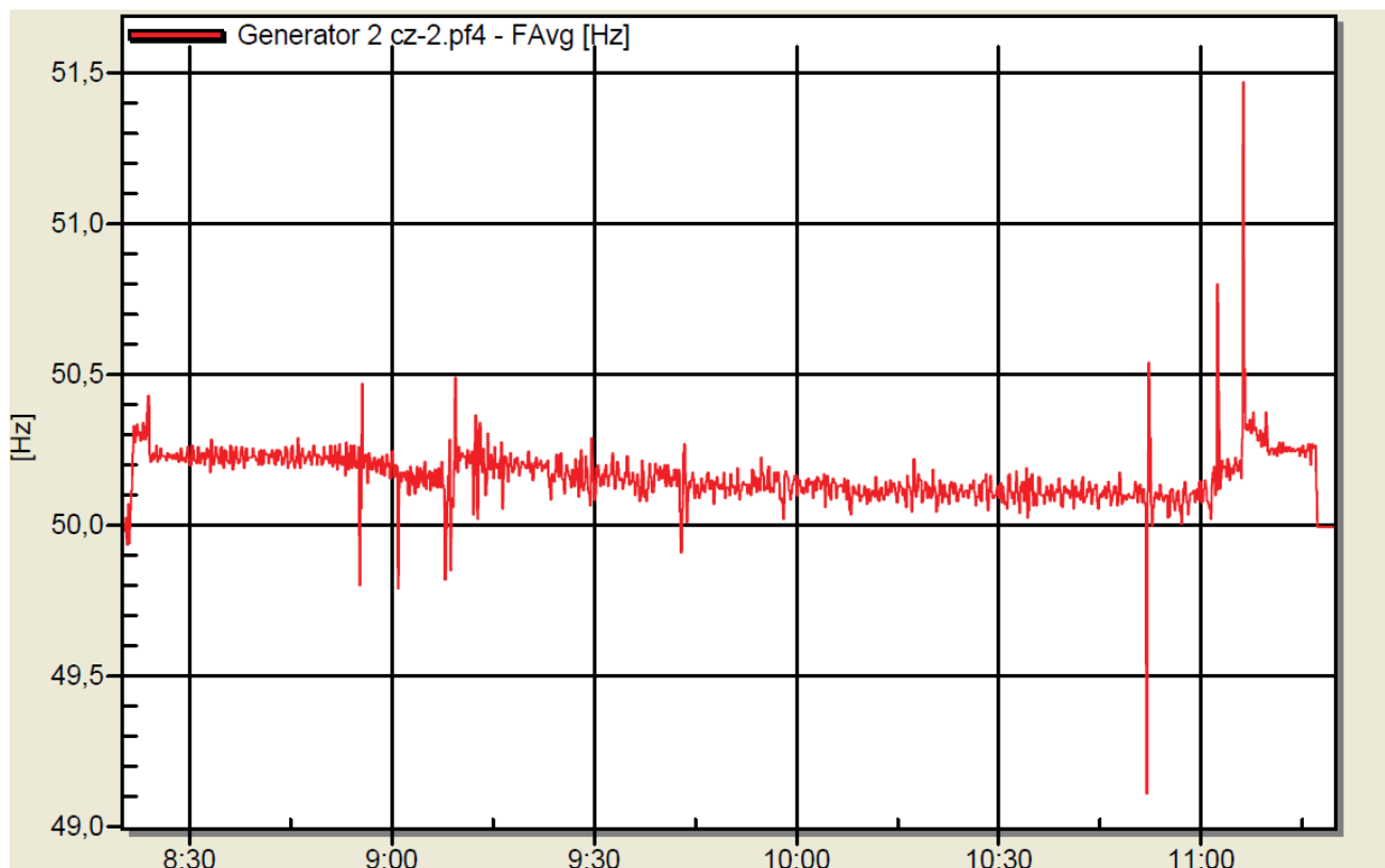
Rys. 7. Zmiany częstotliwości zarejestrowane na zaciskach generatora HG2 w EW Dychów w czasie uruchamiania bloku energetycznego nr 5 w Elektrowni Dolna Odra
