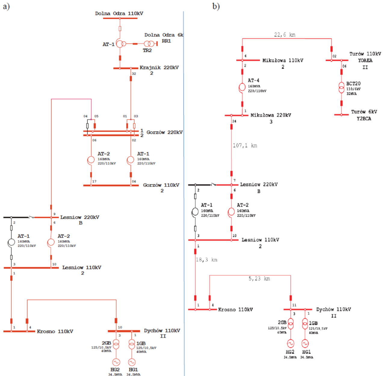
Rys. 1. Uprozczone schematy torów rozruchowych 110 kV i 220 kV z EW Dychów do Elektrowni Dolna Odra (a) oraz z EW Dychów do Elektrowni Turów (b), wydzielone i utworzone podczas dotychczasowych eksperymentów systemowych podania napięcia i mocy rozruchowej.
