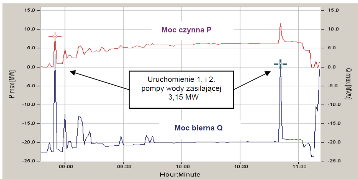
Rys. 6. Zmiany mocy czynnej i biernej w GPZ Dychów w linii 110 kV kierunek Krosno Odrzańskie w czasie uruchamiania bloku energetycznego w Elektrowni Dolna podczas eksperymentu.
