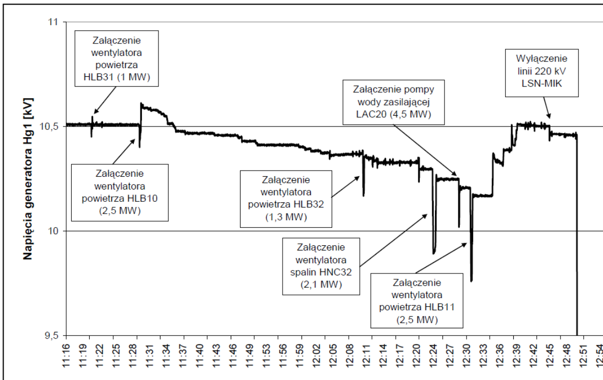
Rys. 9. Zmiany napięcia generatorowego hydrozespołu HG1 w EW Dychów w czasie uruchamiania bloku energetycznego w Elektrowni Turów podczas eksperymentu w 2008 roku
