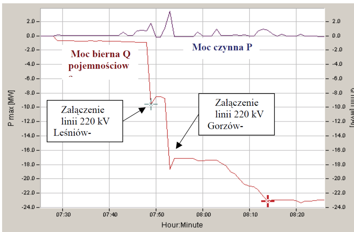
Ryc. 4. Zmiany mocy czynnej i biernej rejestrowane w GPZ Dychów w linii 110 kV kierunku Krosno Odrzańskie w czasie tworzenia toru rozruchowego z EW Dychów do Elektrowni Dolna Odra
