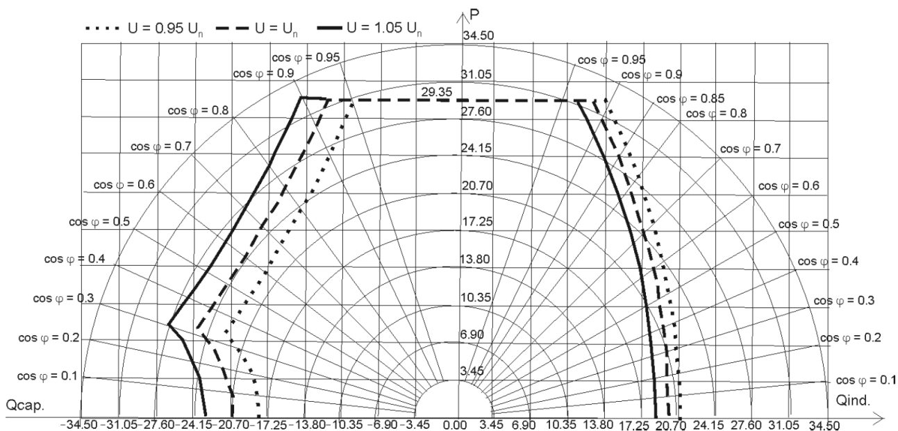
Ryc. 3. Wykres kołowy generatora hydrozespołu HG1
