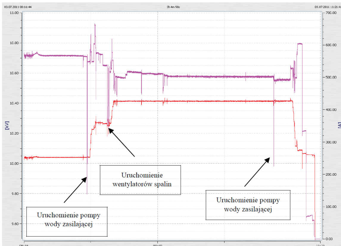
Rys. 5. Zmiany napięcia generatorowego oraz prądu hydrozespołu HG1 w EW Dychów w czasie uruchamiania urządzeń potrzeb własnych bloku energetycznego nr 5 w Elektrowni Dolna Odra
