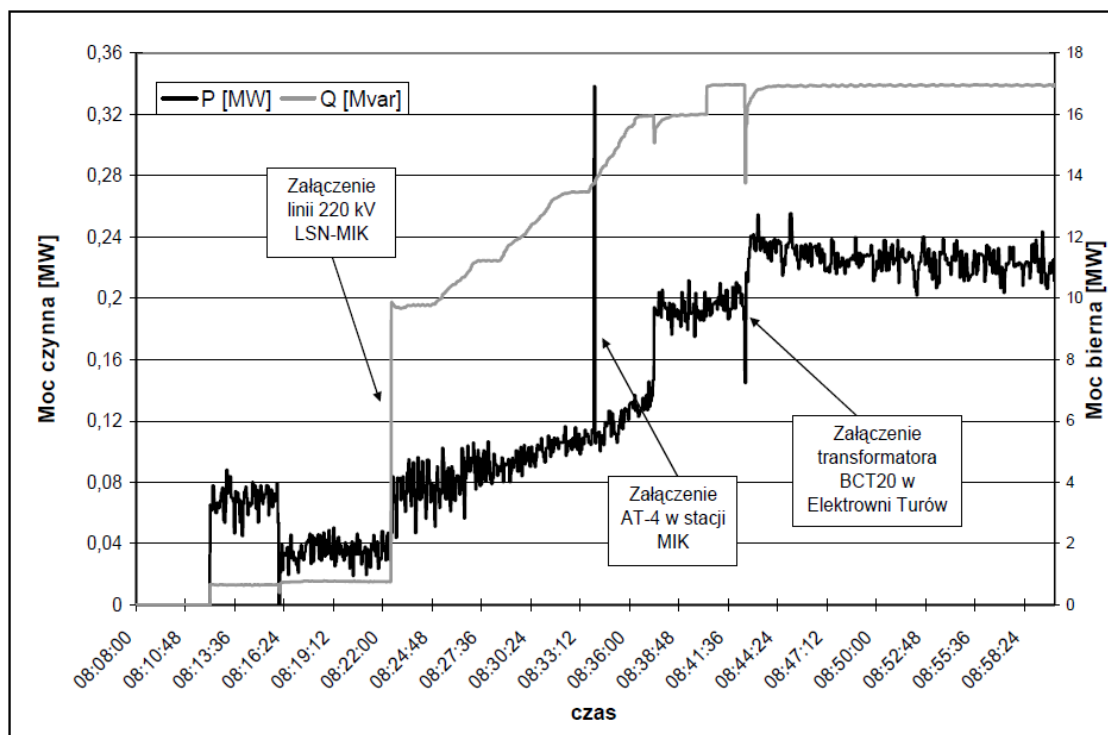
Rys. 8. Moc czynna i bierna w linii 110 kV kierunek Krosno Odrzańskie w czasie tworzenia toru rozruchowego podczas eksperymentu systemowego 2008 roku.
