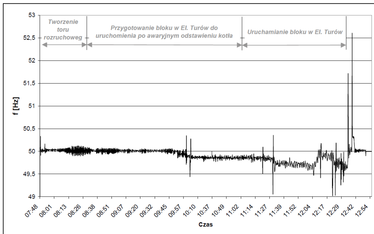
Rys. 11. Zmiany częstotliwości zarejestrowane w EW Dychów w trakcie eksperymentu w 2008 roku
