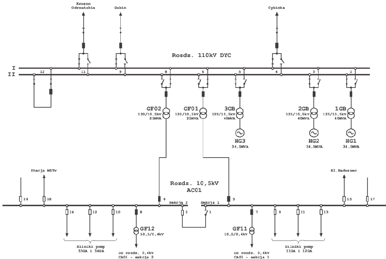
Ryc. 2. Schemat uproszczony GPZ Dychów; rozdzielnia 110 kV (R-110) oraz rozdzielnia 10,5 kV – układ normalny pracy GPZ-u.
